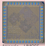
Imperio – UMC65 1x RI5CY
