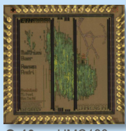
Or10n – UMC180 1x Or10n
